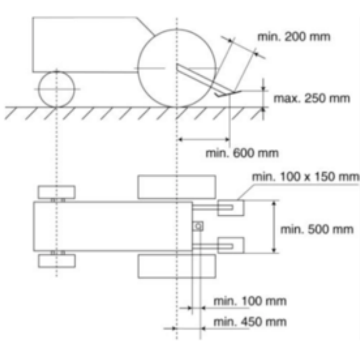
Figuur 1 : Steigerbegrenzer
